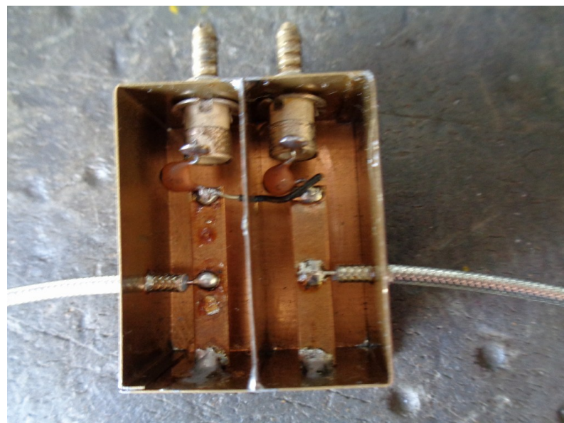
1300MHz BPF
