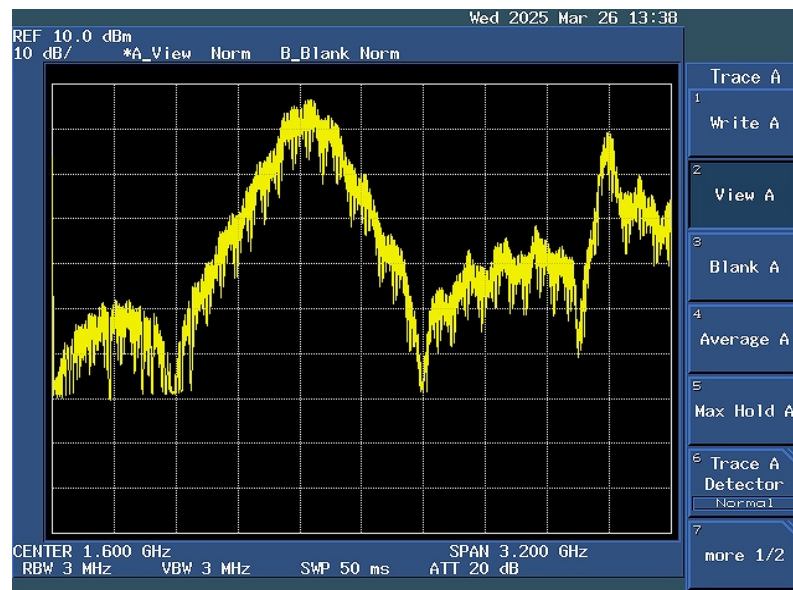
周波数特性(SGで10MHz step max hold測定)
