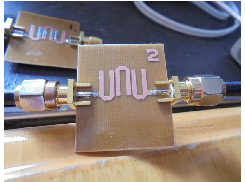
写真2. 5032MHz BPF
