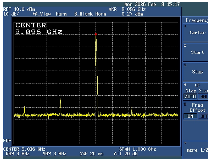
写真3. 対策後の9096MHz
