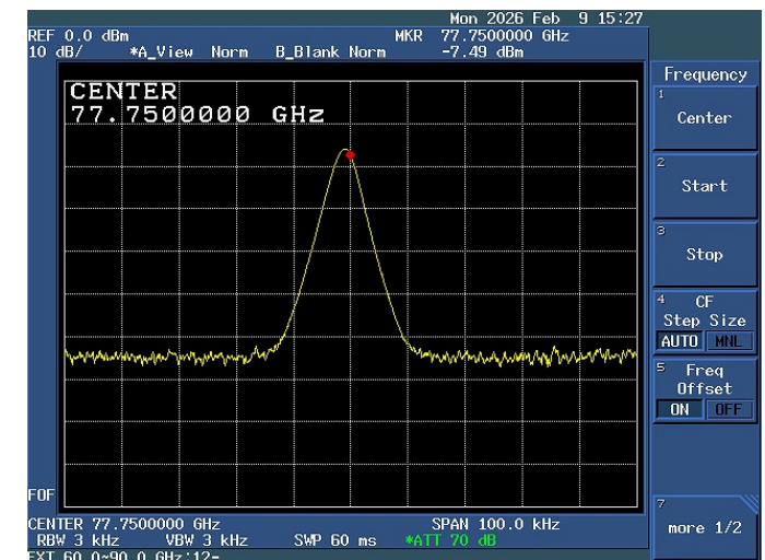
写真4. 対策後の77GHz出力
