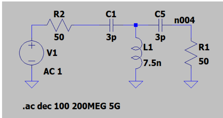
図1. HPF回路
