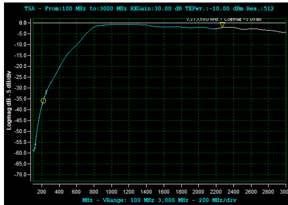
図2. 実測結果
