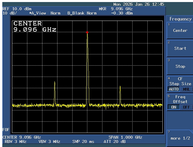
写真2. 対策前の9096MHz
