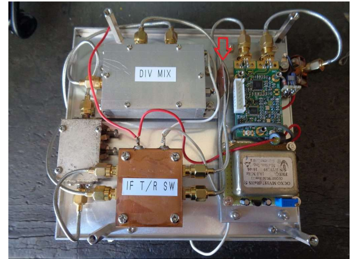
写真1. HPF挿入箇所
