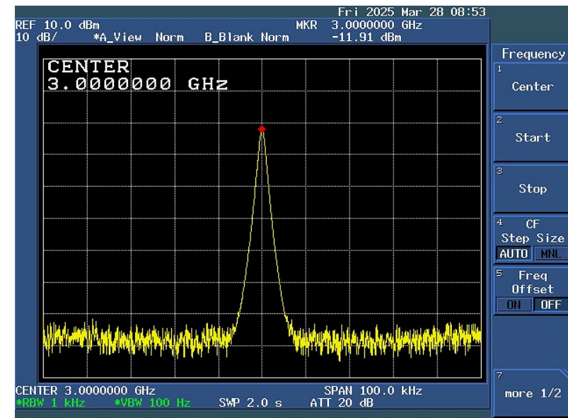
図8. C/Nも悪くはない？
