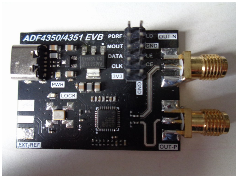
図1. ADF4350評価基板
