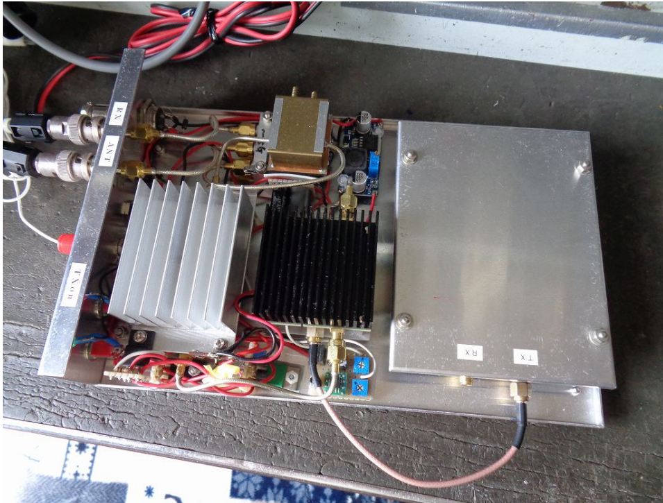
DATV 送信機
