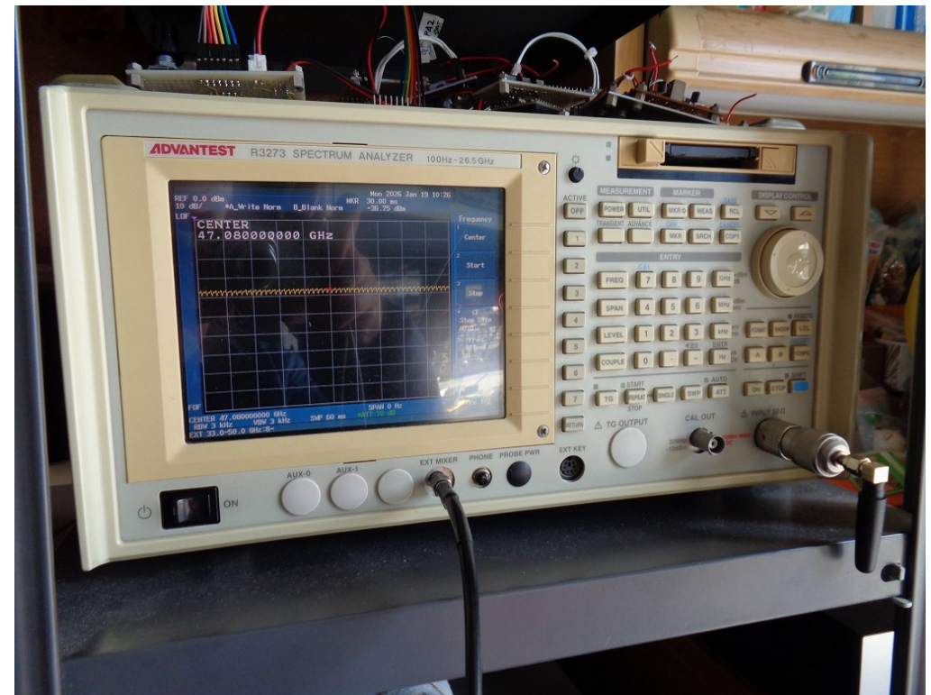
写真2. SPANは0Hz
