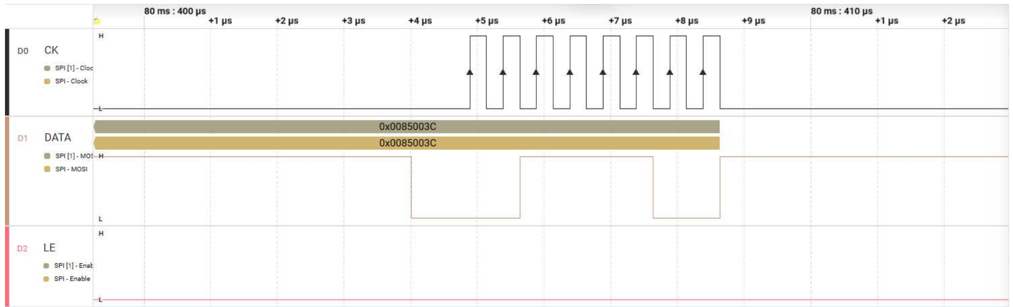
図2. R4付近のSPI波形拡大
