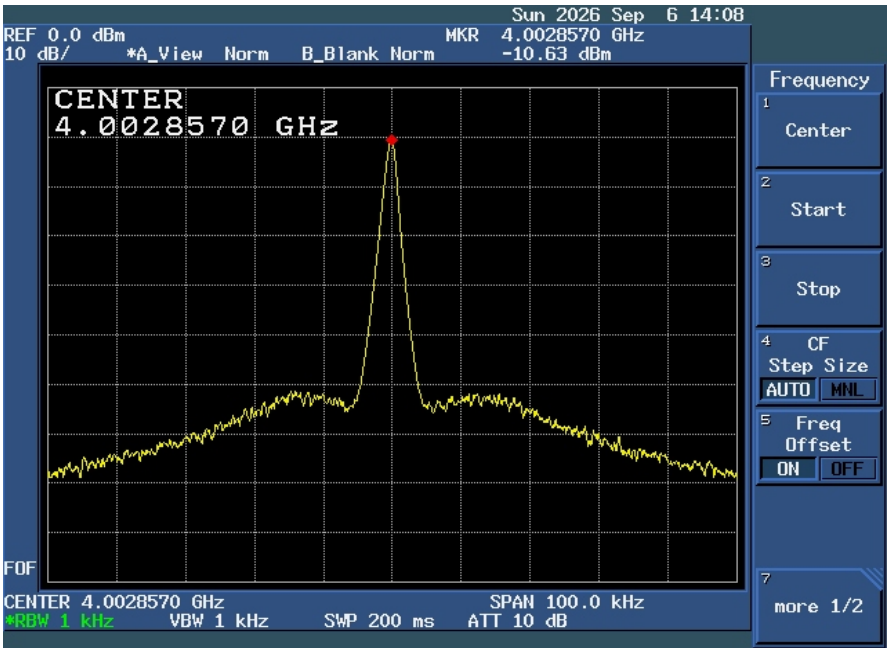
写真2. 4003MHz出力(C/Nについての考慮無し)
