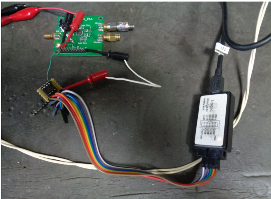
写真1. SPI波形観測
