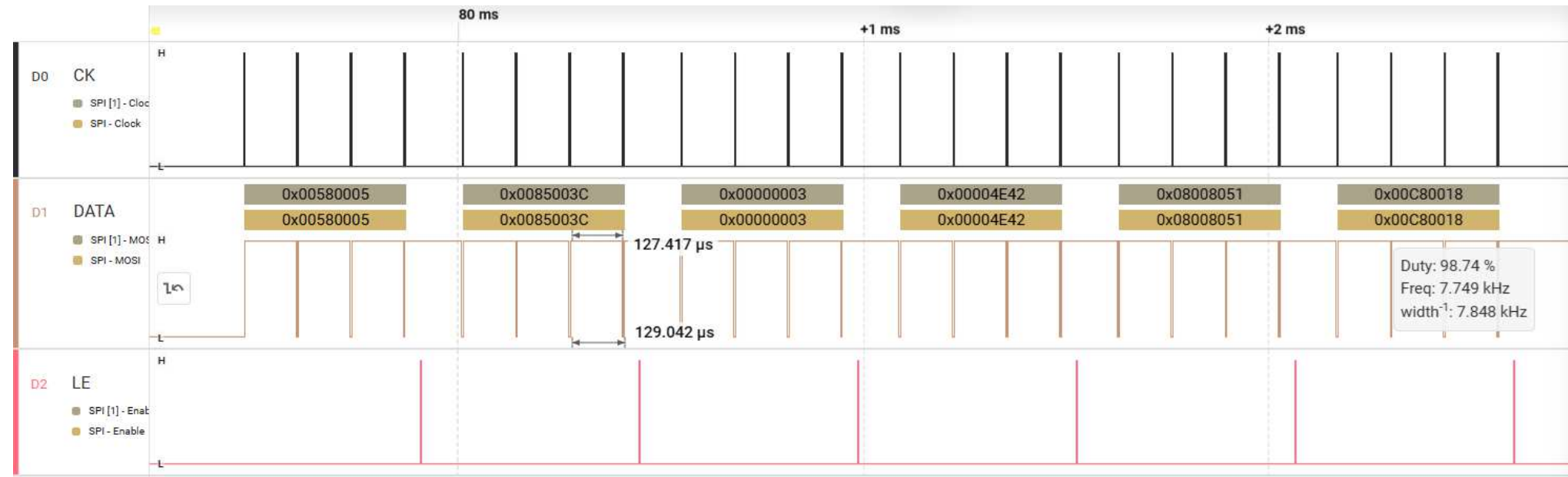
図1. SPI波形全体
