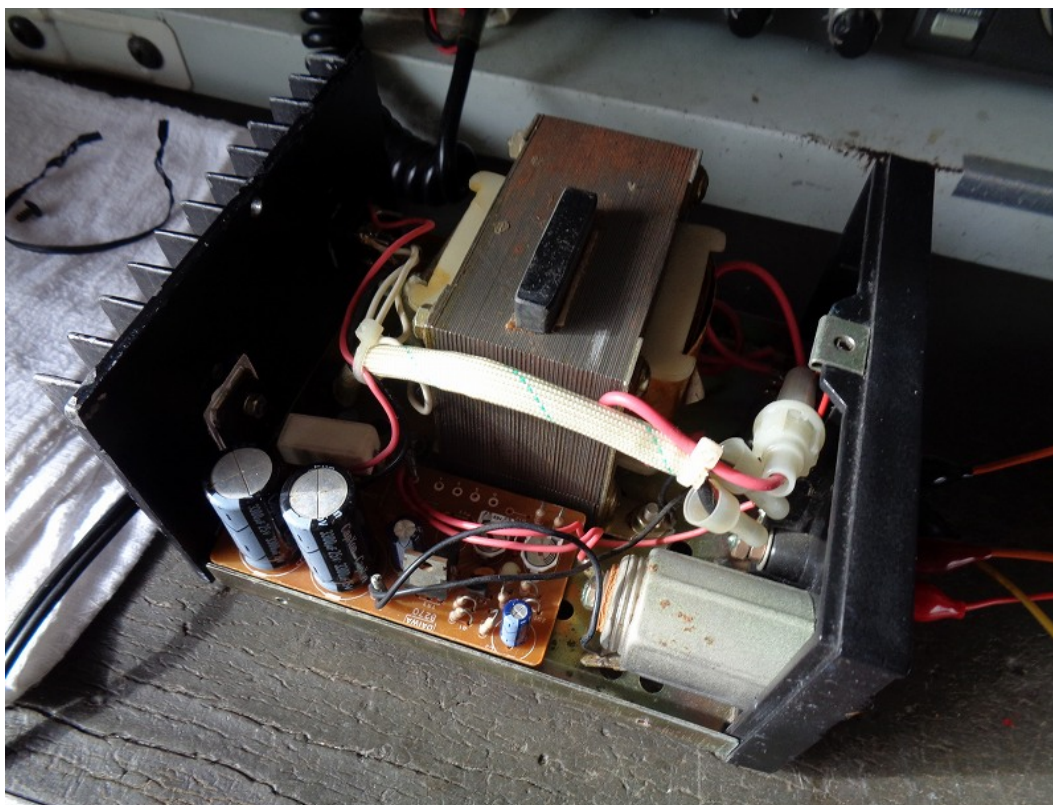
図1. PS-55T外観
