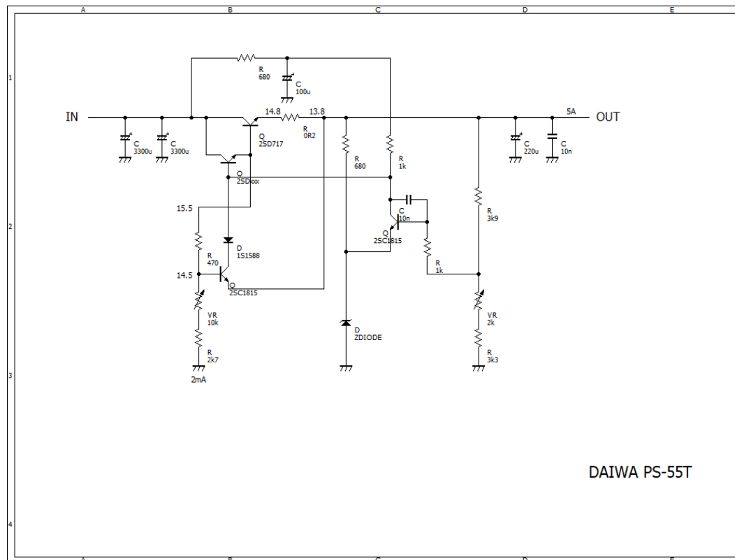
図2. PS-55T 回路図
